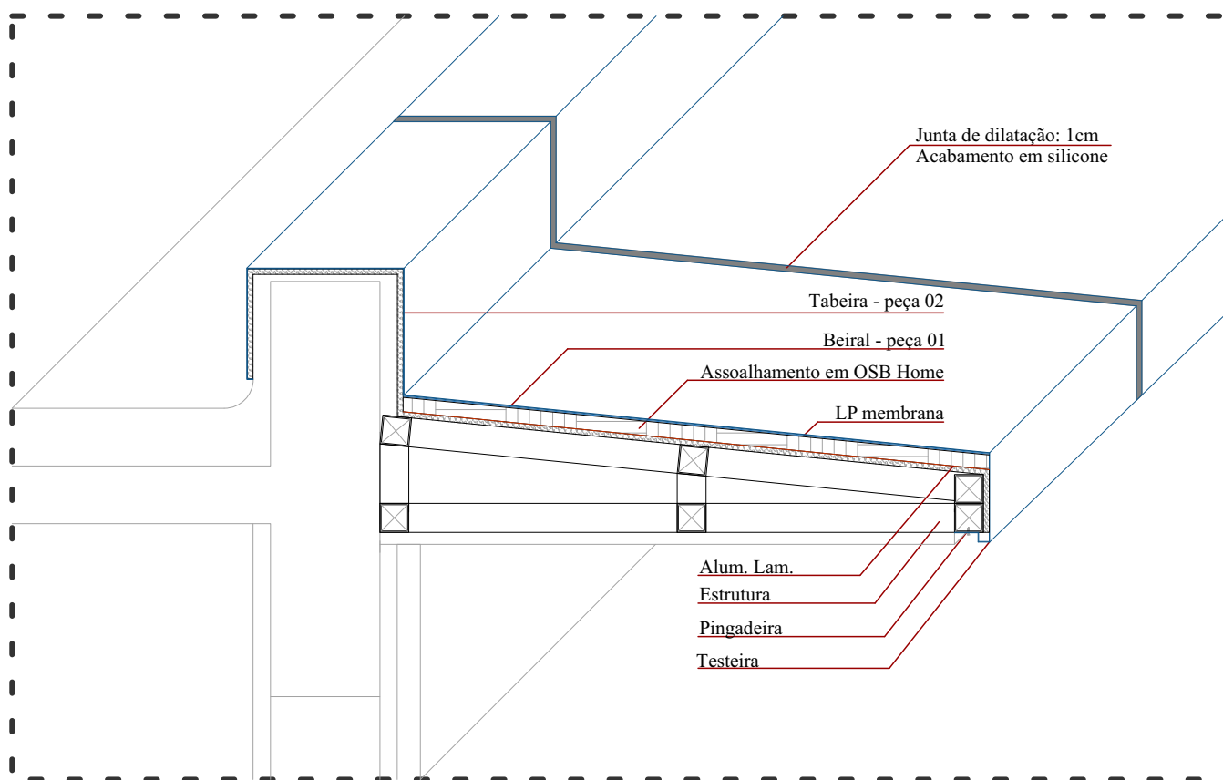
Corte Transversal | Tipo
